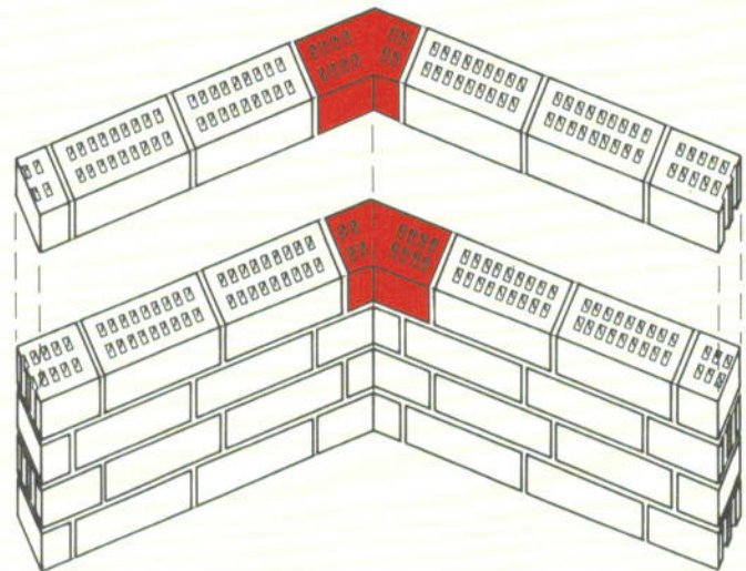
Innenecken- ausbildung 45°
