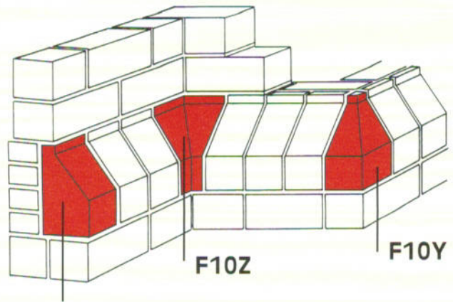
Eckenausbildungen
